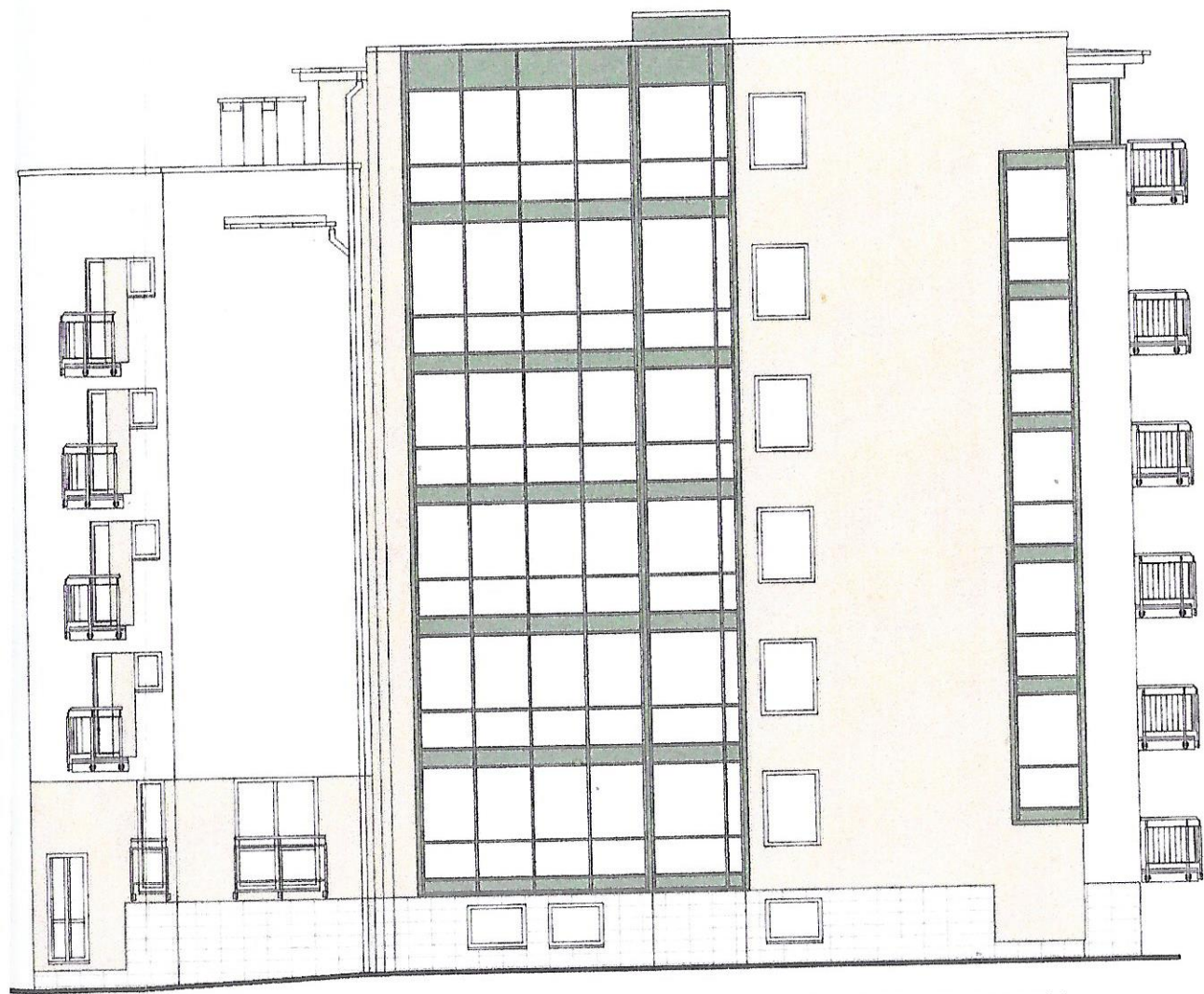
ELEVACJA WSCHODNIA
